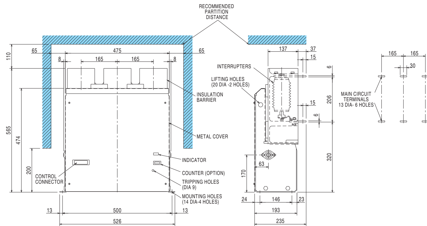
Fig. 13 Types CV-10HA(L)/CV-10HB(L)
