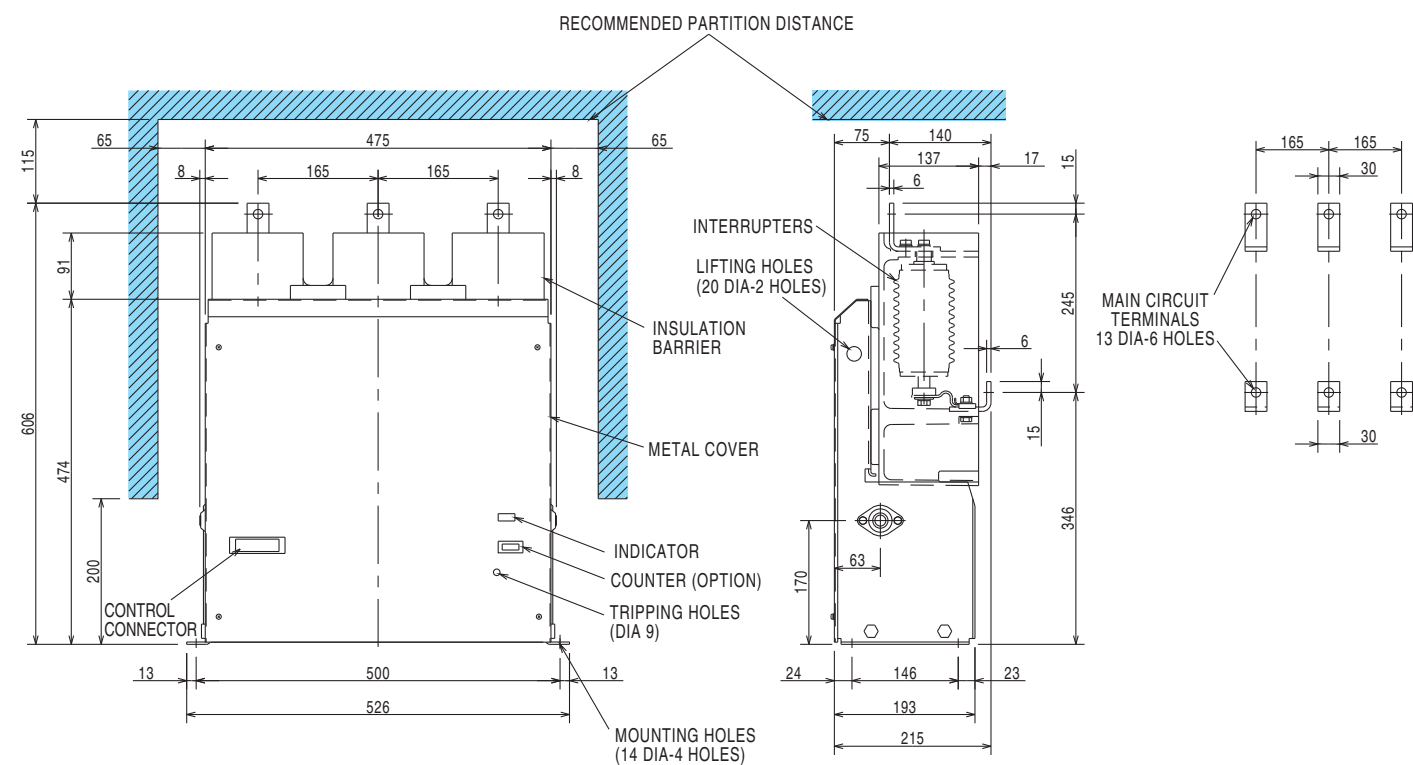
Fig. 14 Types CV-10HA(L)-1/CV-10HB(L)-1
