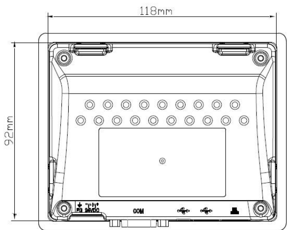
Вид сзади
