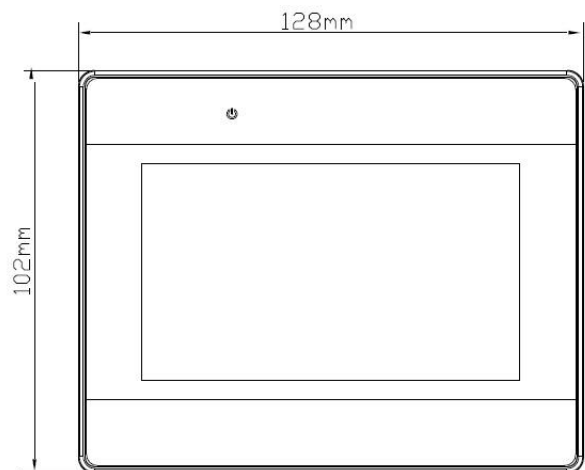
Вид спереди
